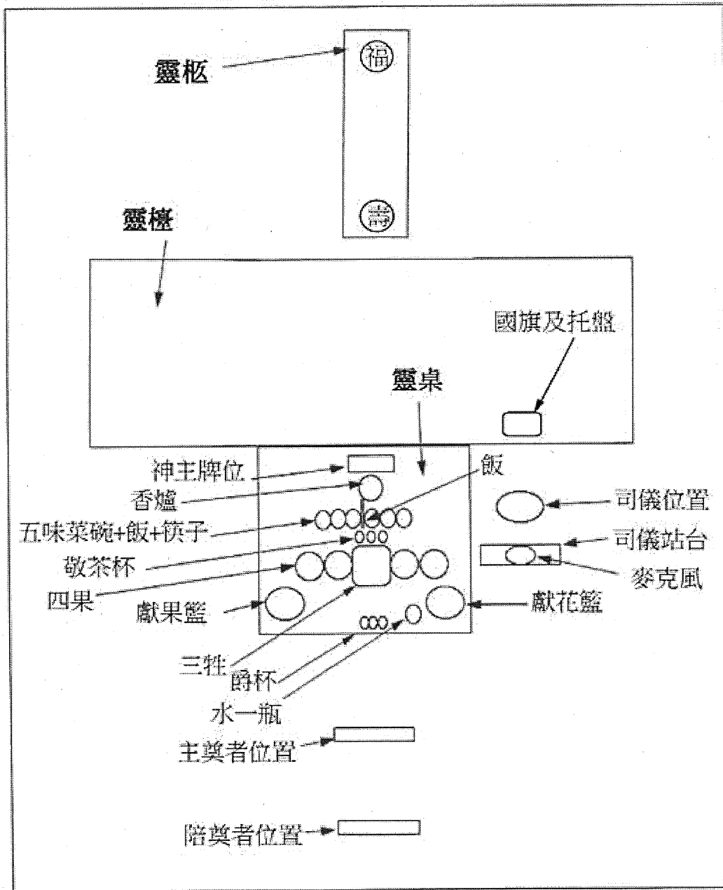
附圖三、情境3-懇辭花籃之奠禮會場布置標準圖(使用獻花籃)
