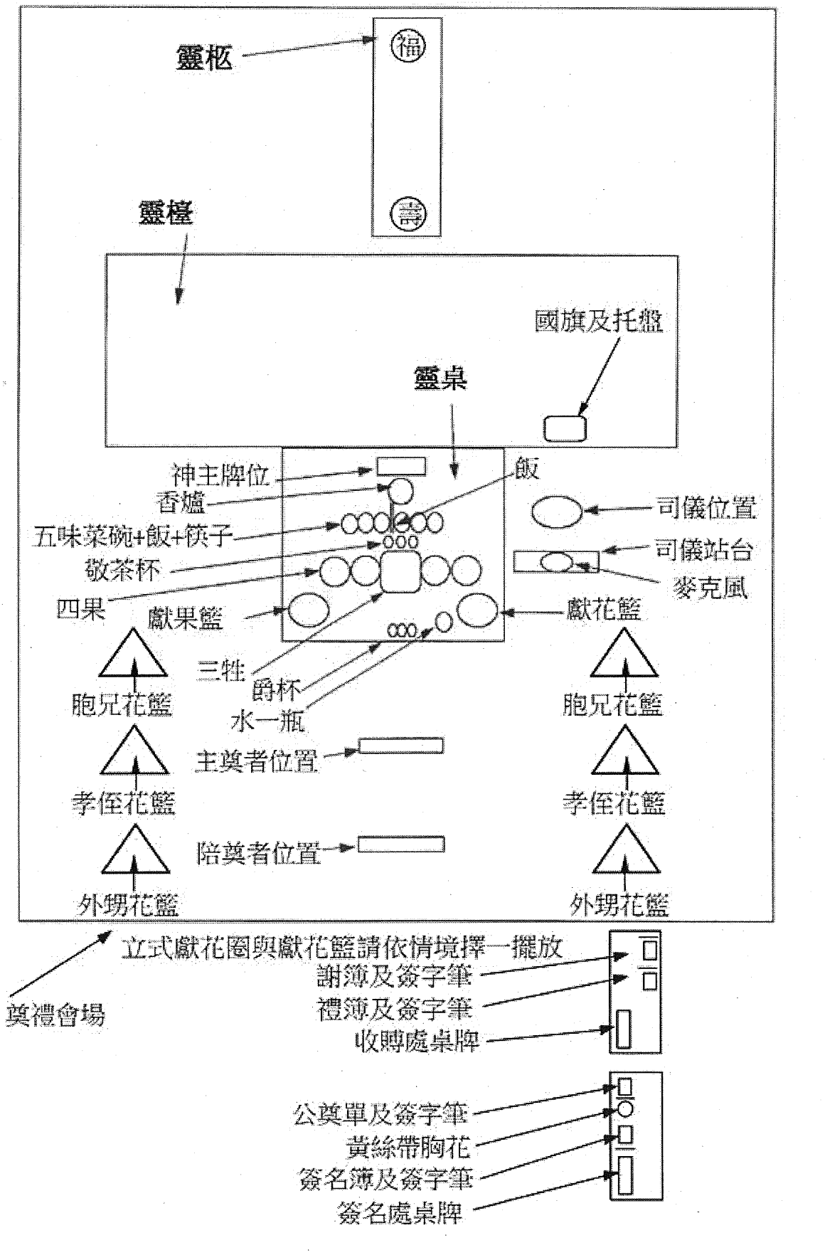
附圖一、情境 1-一般模式之奠禮會場布置標準圖(使用獻花籃)
